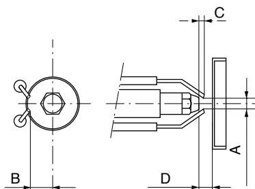
N 50/2 - N 75/2
