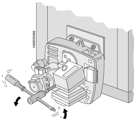
Abb. B. Durch Lösen des Befestigungszapfens der Platte kann der Brenner geöffnet werden. Nun sind zugänglich: Lüfterrad, Öldüse, Elektroden und Ölvorwärmer.
