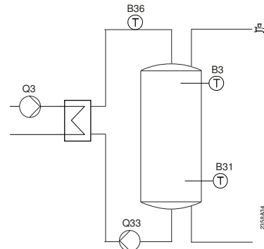
Serbatoio ACS con scambiatore di calore esterno, pompa di ricarica, pompa del circuito intermedio
