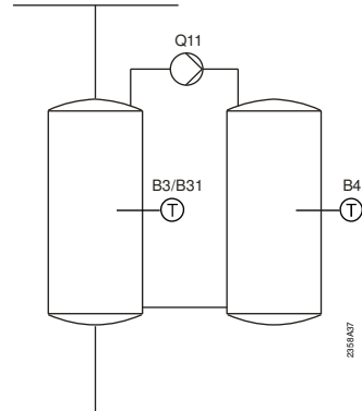
Trasferimento ricarica del serbatoio
