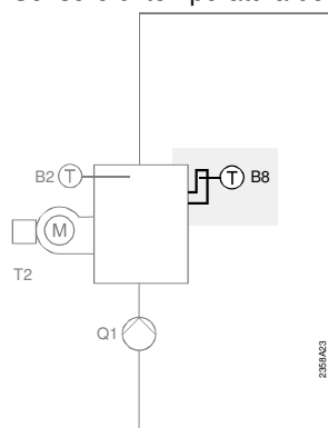
Sensore di temperatura del condotto del gas
