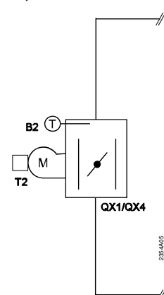
Modulazione a 3 punti 0...10 V
