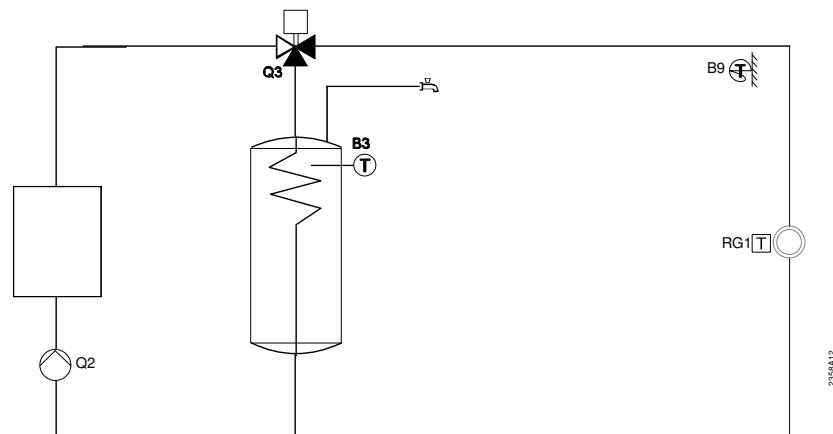
Riscaldamento ACS con valvola deviatrice
