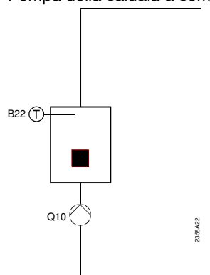
Pompa della caldaia a combustibile solido
