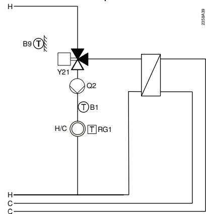
Valvola deviatrice per il raffreddamento
