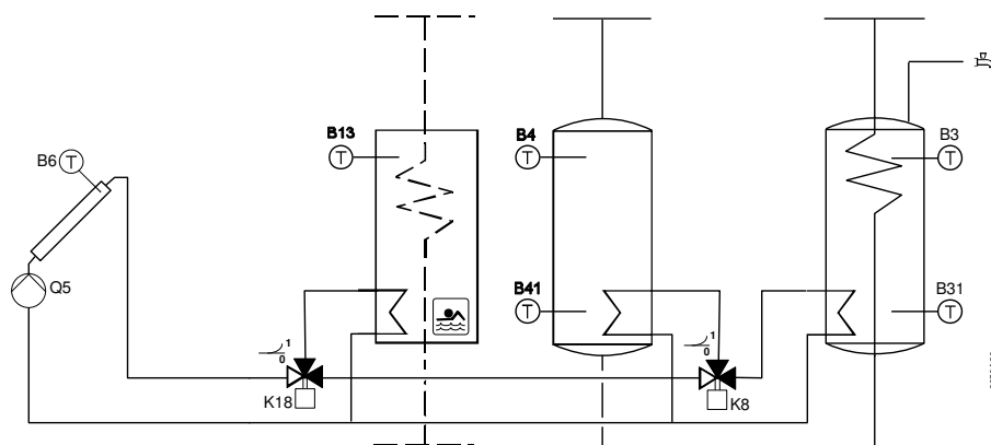
Ricarica solare del serbatoio e della piscina mediante valvole deviatrici con 1 collettore
