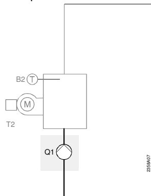
Pompa della caldaia
