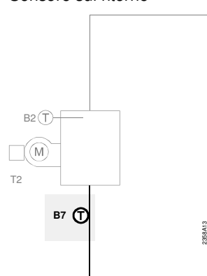
Sensore sul ritorno
