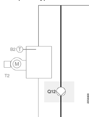
Pompa di bypass
