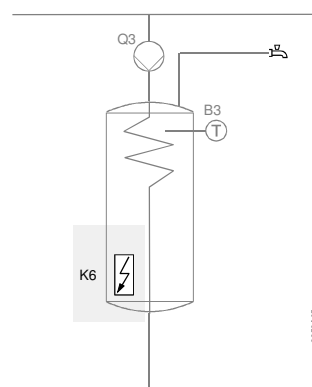
Riscaldatore elettrico ad immersione ACS
