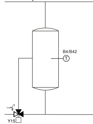
Ricarica parziale del serbatoio
