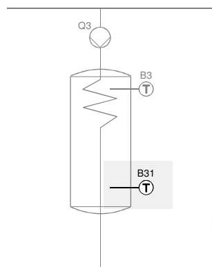
2° sensore ACS
