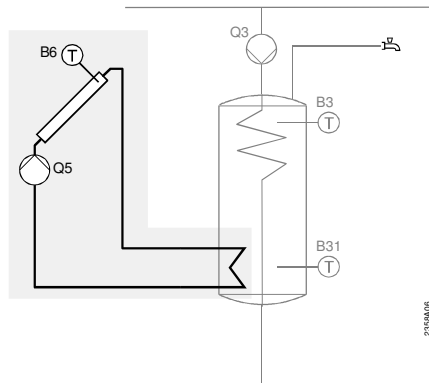
Pompa del collettore di ricarica ACS, sensore del collettore
