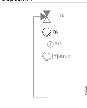
2° valvola miscelazione circuito di riscaldamento
