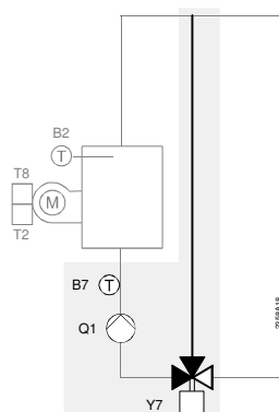
Regolatore della temperatura sul ritorno
