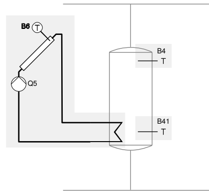
Ricarica del serbatoio di riserva
