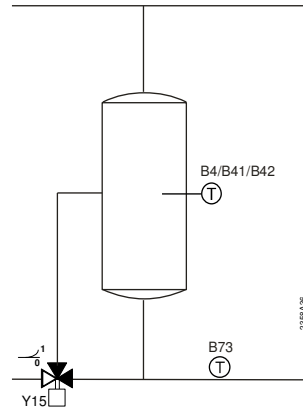
Deviazione del ritorno
