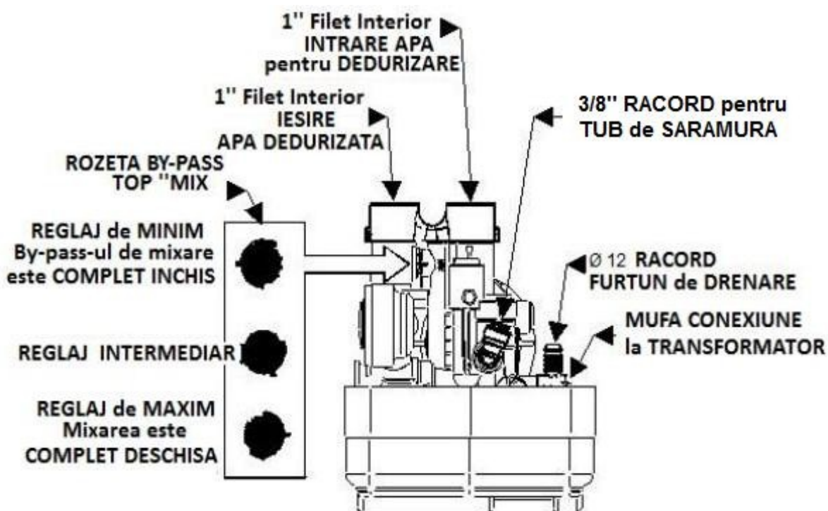
Fig. 8 SCHEMA de RACORDARE HIDRAULICA
